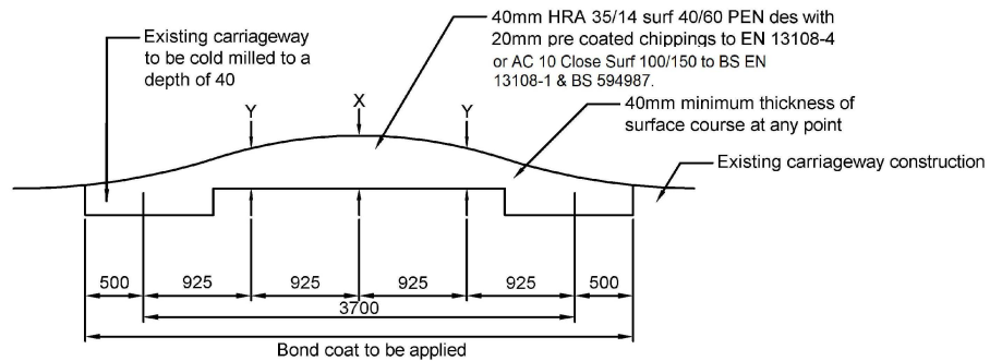
LONGITUDINAL SECTION
