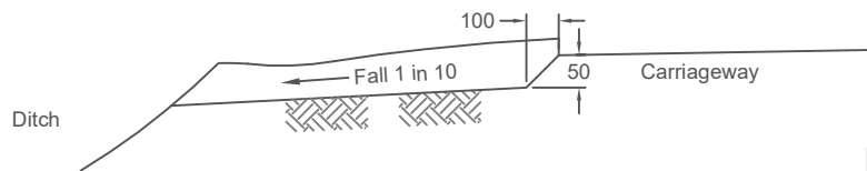
SECTION A-A
